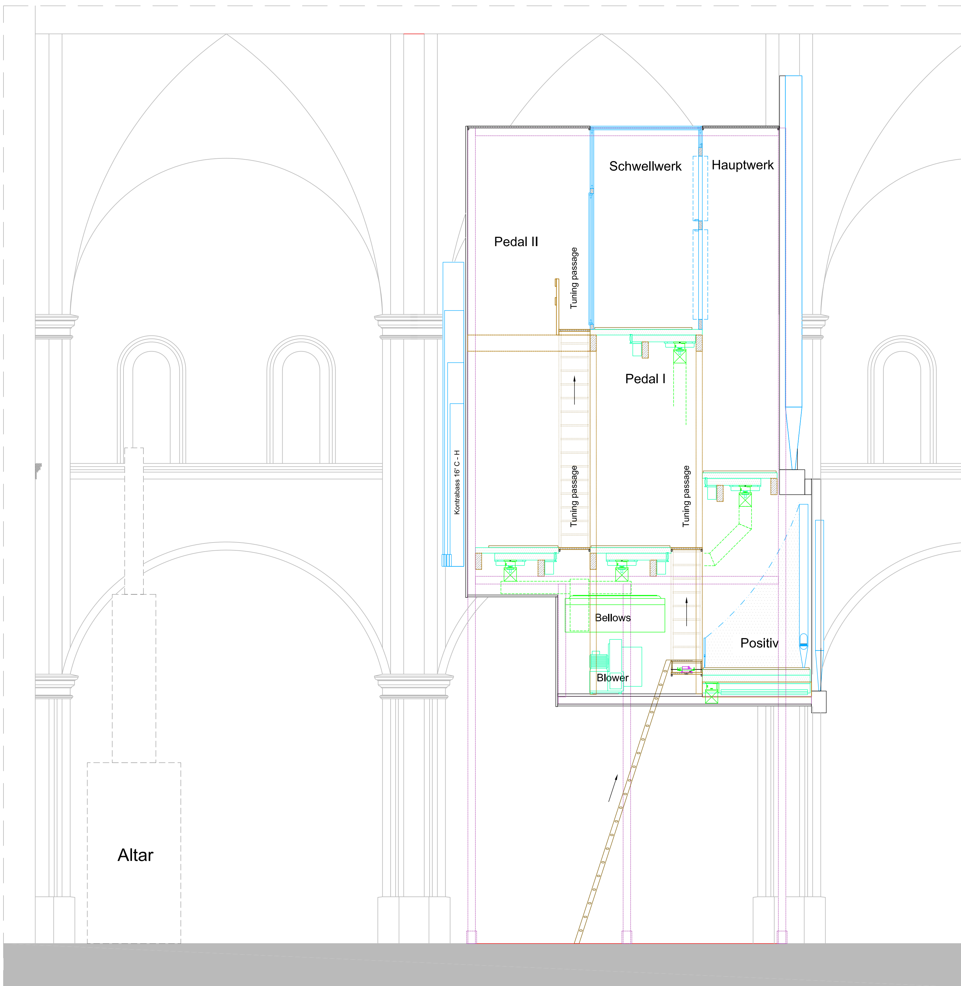
Section E - E
